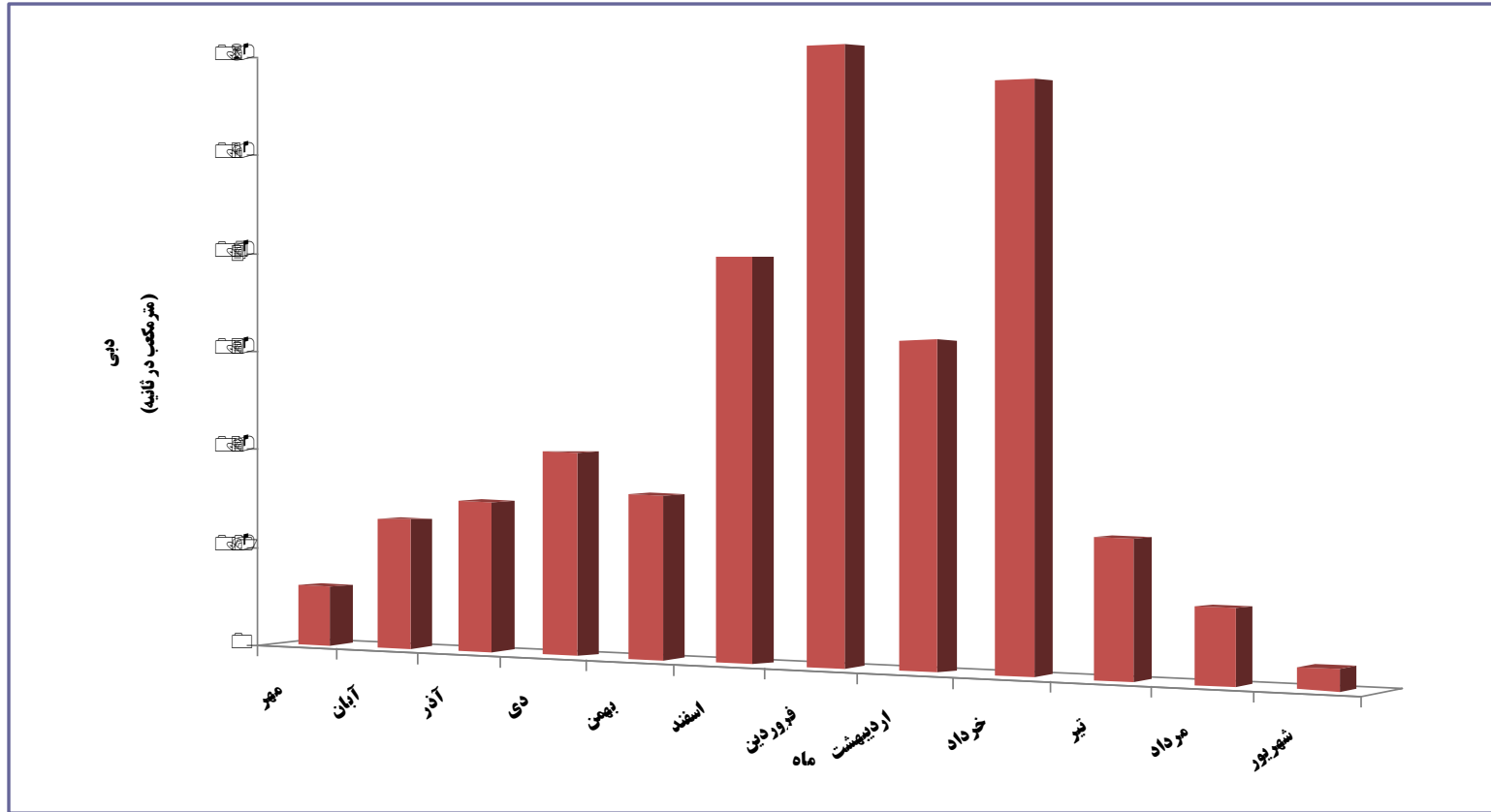
نمودار ( ۲۲-۲ ): رزیم آبدهی متوسط ماهیانه رودخانه گرمی جای در محل ایستگاه آب سنجی گرمی (برحسب مترمکعب در ثانیه)
