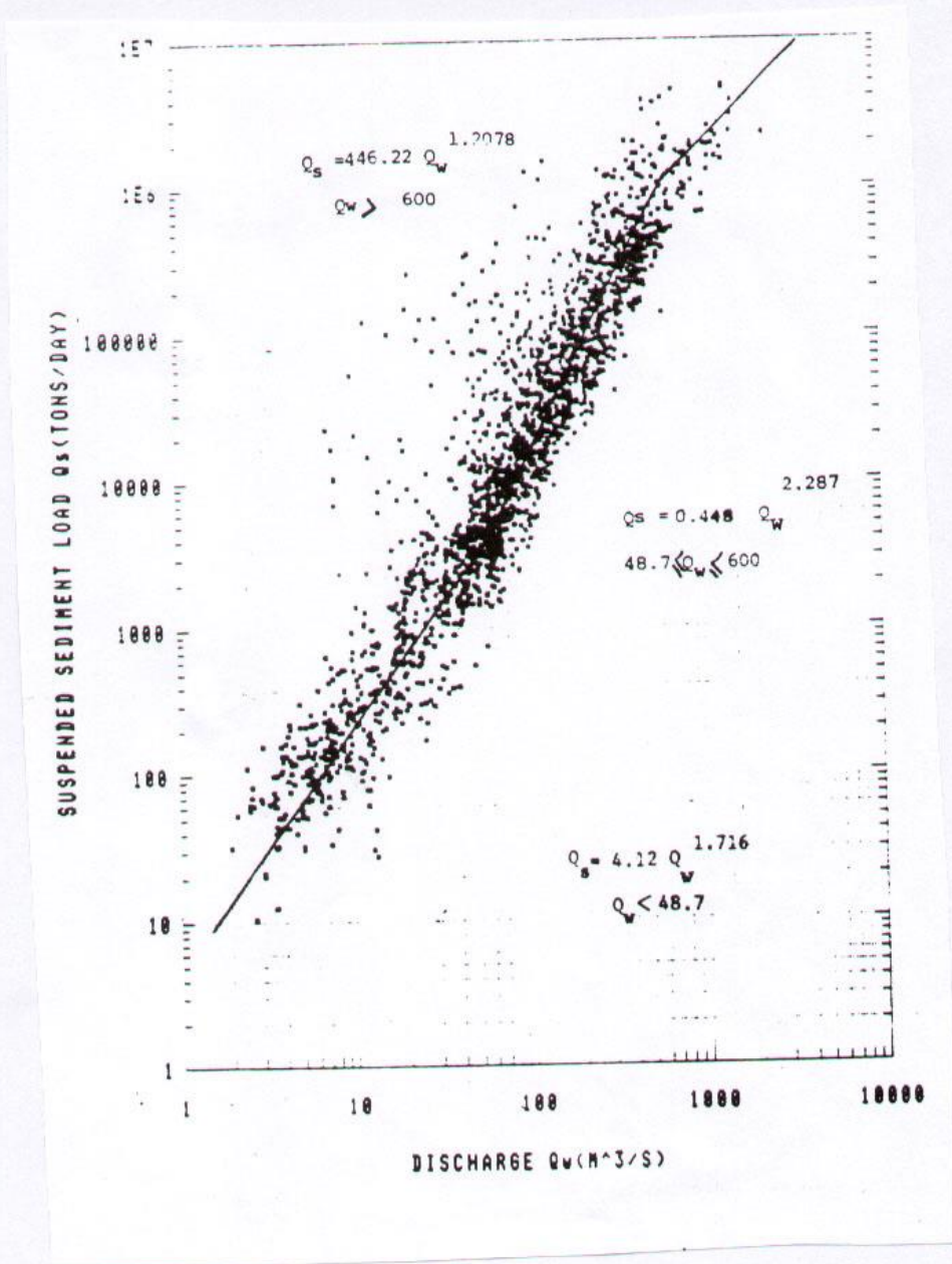
نمودار (۳۱-۲): تغییرات شدت رسوبدهی رودخانه قزل اوزن در ایستگاه گیلوان نسبت به تغییرات آبدهی
