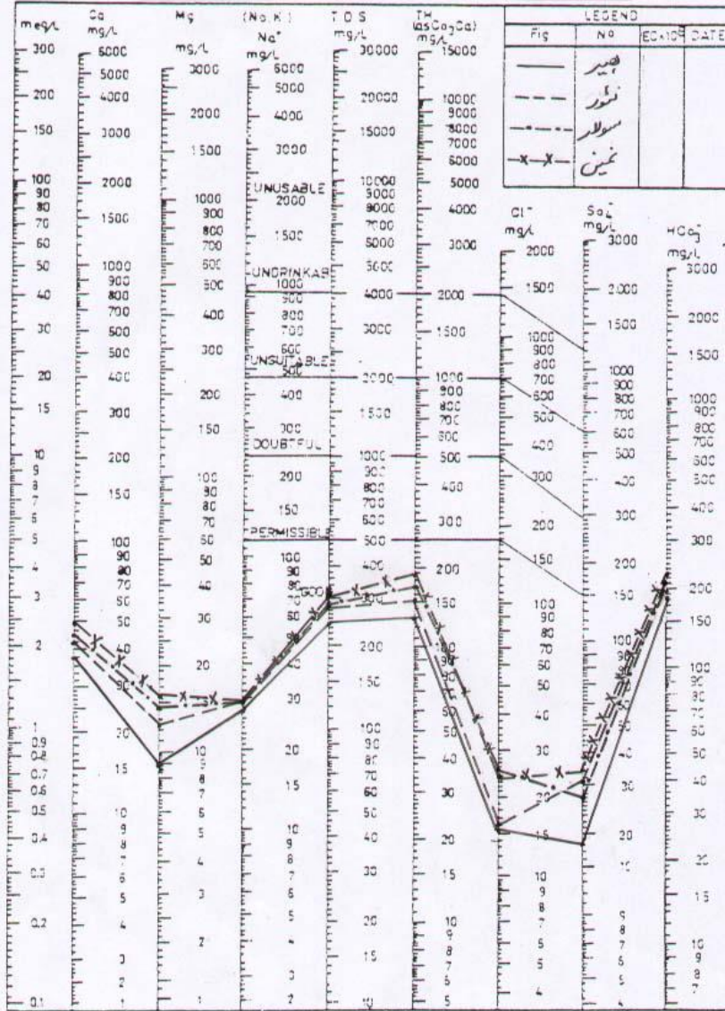
نمودار (۲-۲۸): دیاگرام شولر رودخانه های هیرجای، سولارچای و نمین چای
