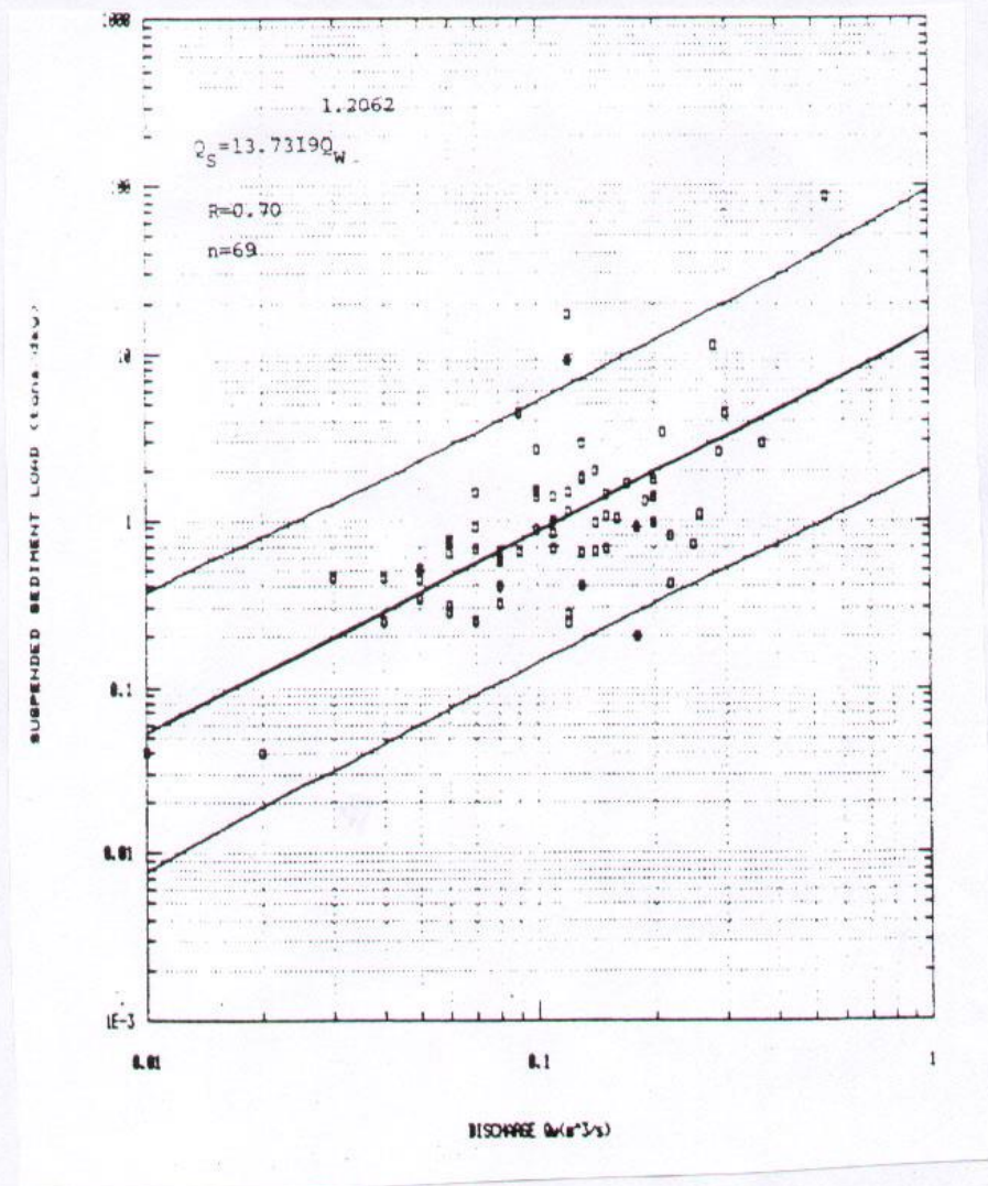
نمودار (۲-۳۲): تغییرات شدید رسوبدهی رودخانه لای چای در ایستگاه لای نسبت به تغییرات آبدهی
