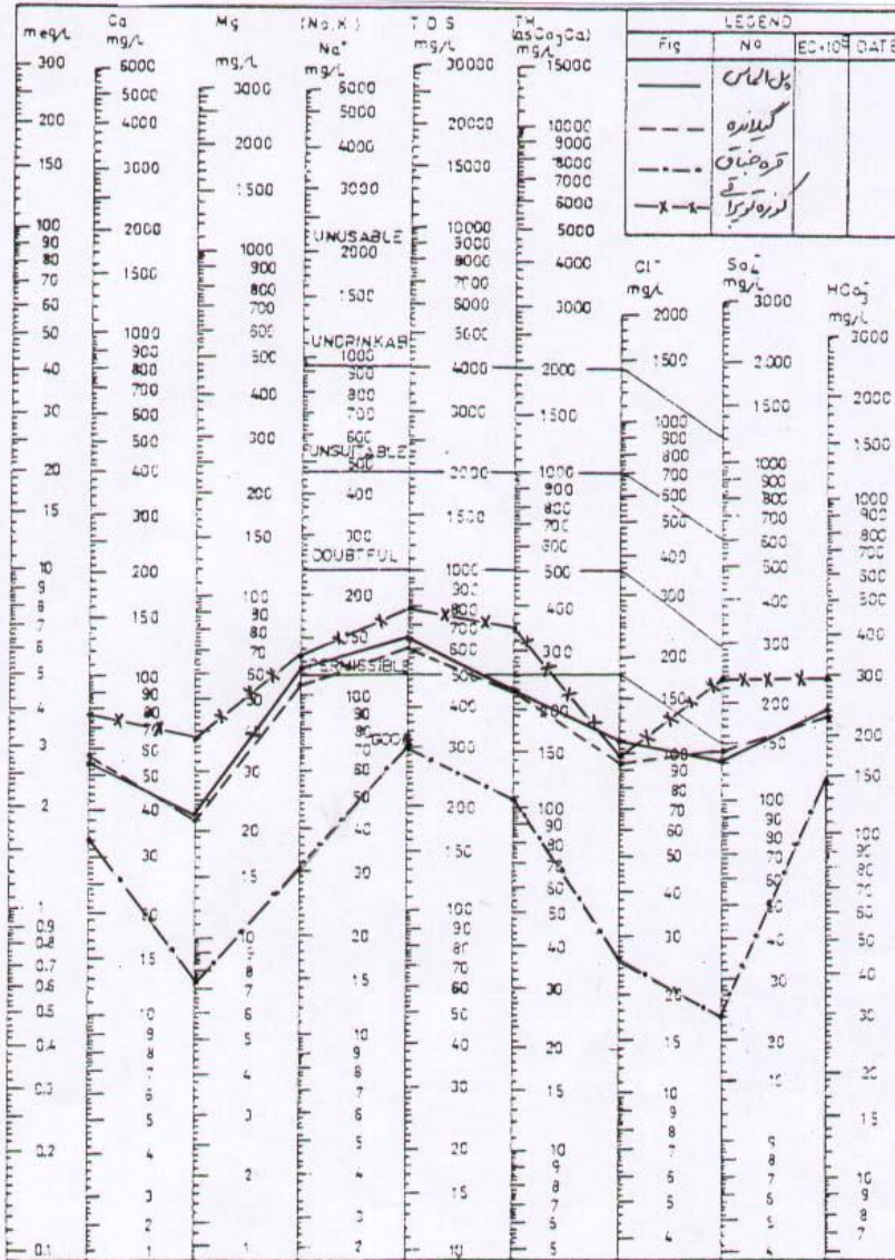
نمودار (۲۶-۲): دیگرام شولر رودخانه های بالیخوچای، قره سو و قوری جای
