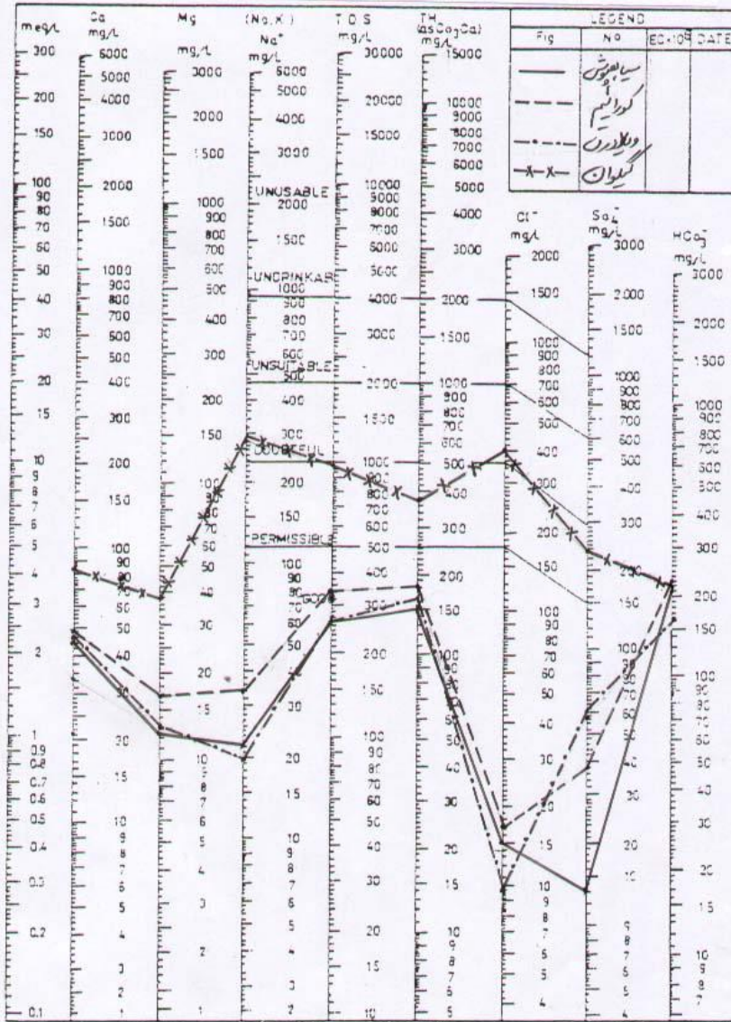
نمودار (۳۰-۲): دیاگرام شولر رودخانه های فوری جای، بایلوخجای و قزل اوزن
