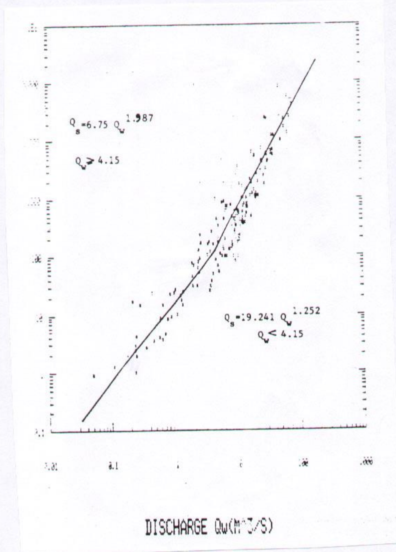
نمودار (۳۶-۲): تغییرات شدت رسوبدهی رودخانه قره سو در ایستگاه دوست بیگلو نسبت به تغییرات آبدهی
