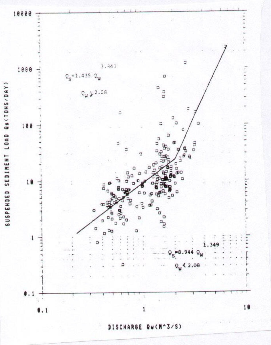
نمودار (۳۳-۲): تغییرات شدت رسوبدهی رودخانه نیرجای در ایستگاه نیر نسبت به تغییرات آبدهی
