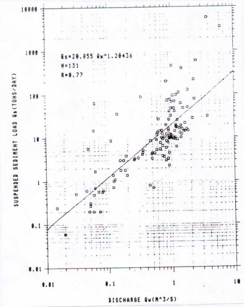
نمودار (۳۵-۲): تغییرات شدت رسوبدهی رودخانه خیاوچای در ایستگاه پل سلطانی نسبت به تغییرات آبدهی
