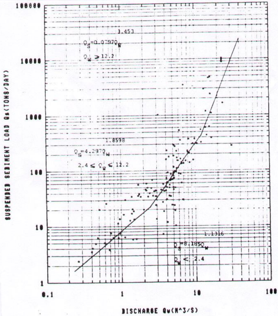
نمودار (۳-۳۴): تغییرات شدت رسوبدهی رودخانه بالیخوجای در ایستگاه پل الماس نسبت به تغییرات آبدهی
