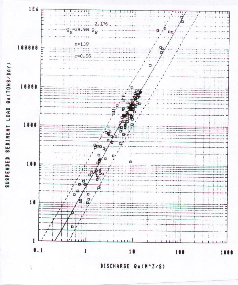
نمودار (۳۹-۲): تغییرات شدت رسوبدهی رودخانه بارون جای در ایستگاه بارون نسبت به تغییرات آبدهی
