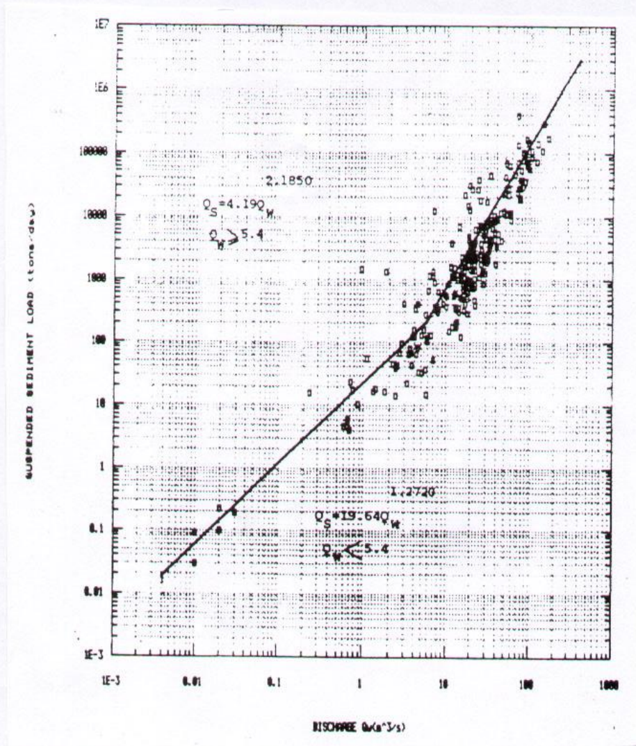
نمودار (۲-۳۸): تغییرات شدت رسوبدهی رودخانه دره رود در ایستگاه بوران نسبت به تغییرات آبدهی
